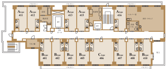
間取り 5F
