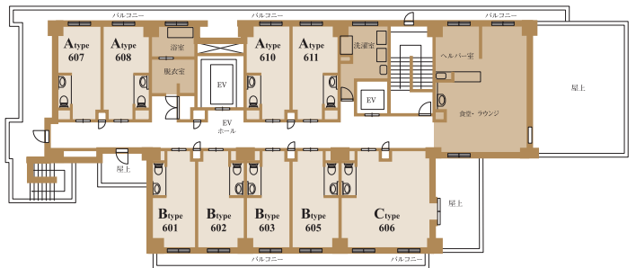
間取り 6F
